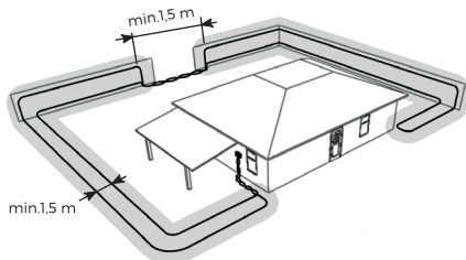
Typ 3: Podział działki na dwie części za pomocą jednej pętli. Podział działki można również wykonać poprzez podłączenie 2 równoległych pętli z jednego generatora. Uwaga: W drugim przypadku w przypadku przerwania jednej pętli generator nie zgłosi błędu.
