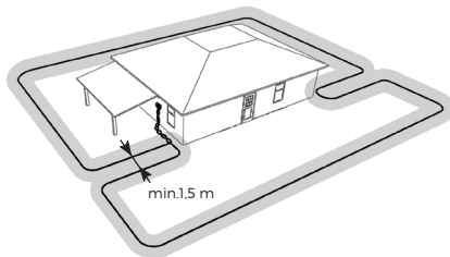
Tipo 3: Divisione del terreno in due parti mediante un unico circuito. La divisione del terreno può essere effettuata anche collegando due circuiti paralleli da un unico generatore. Attenzione: nel secondo caso, in caso di interruzione di uno dei circuiti, il generatore non segnalerà alcun errore.
