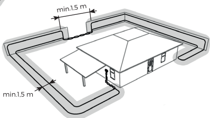
Typ 3: Rozdělení pozemku na dvě části pomocí jedné smyčky. Rozdělení pozemku je možno provést i zapojením 2 paralelních smyček z jednoho generátoru. Pozor: V druhém případě se při přerušení jedné smyčky neohlásí chyba na generátoru.
